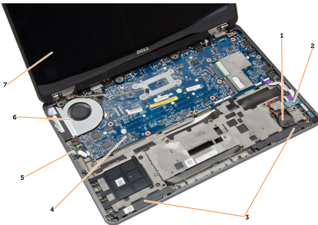
Figur 2. Set indvendigt – Front
